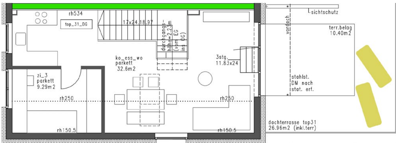
DACHGESCHOSS
