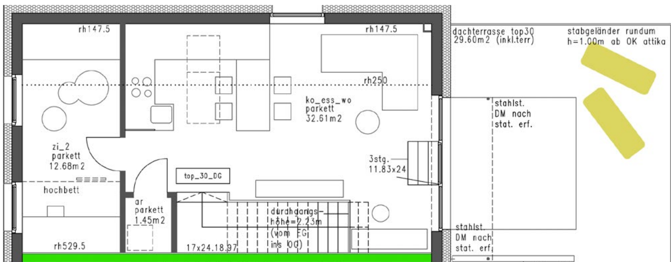
DACHGESCHOSS
